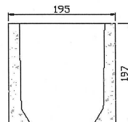
SECCIÓ A-A'
